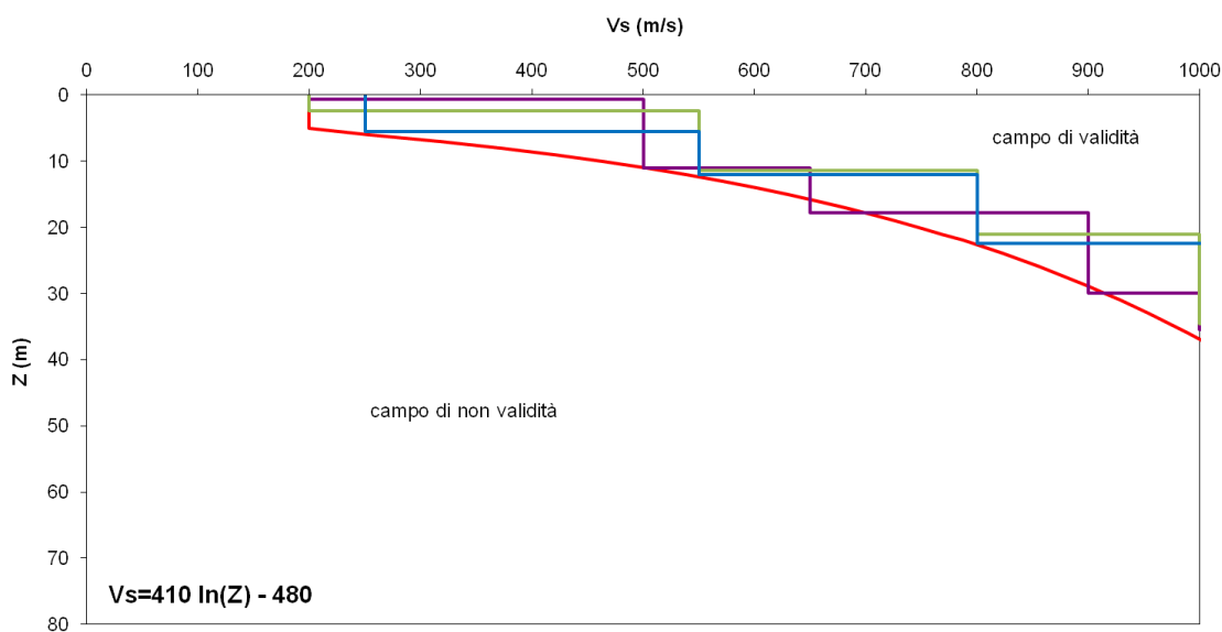
SCHEDA LITOLOGIA GHIAIOSA Andamento dei valori di Vs con la profondità
